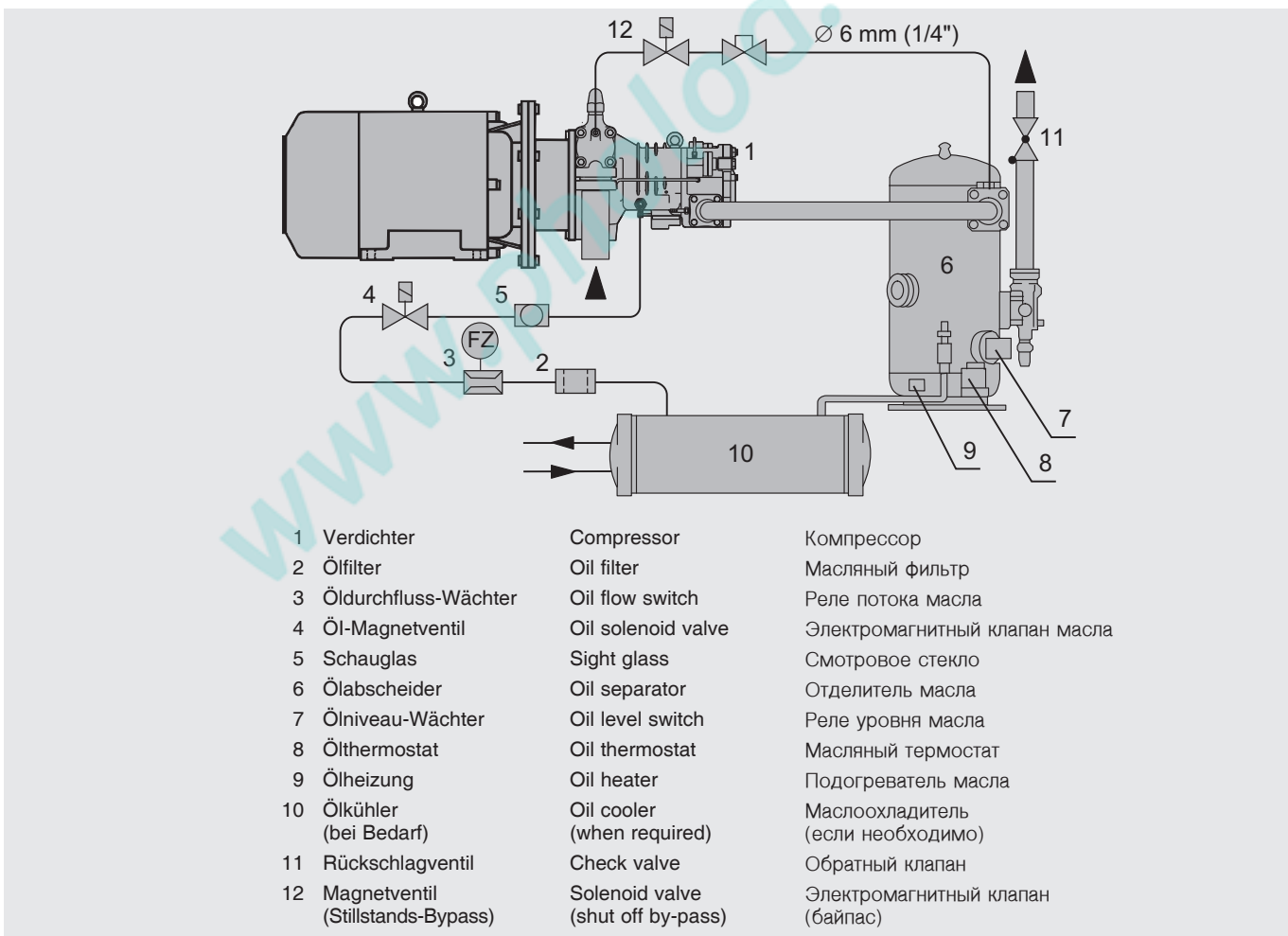
Abb. 6 Schmierölkreislauf
